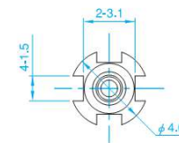
图：ASC-PSB10-2t
