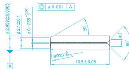
图：ASC-PSB10-2t
