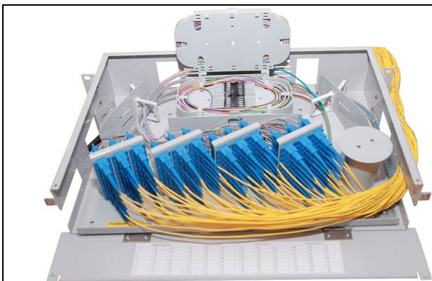
Đầu nhảy dây quang đến thiết bị
