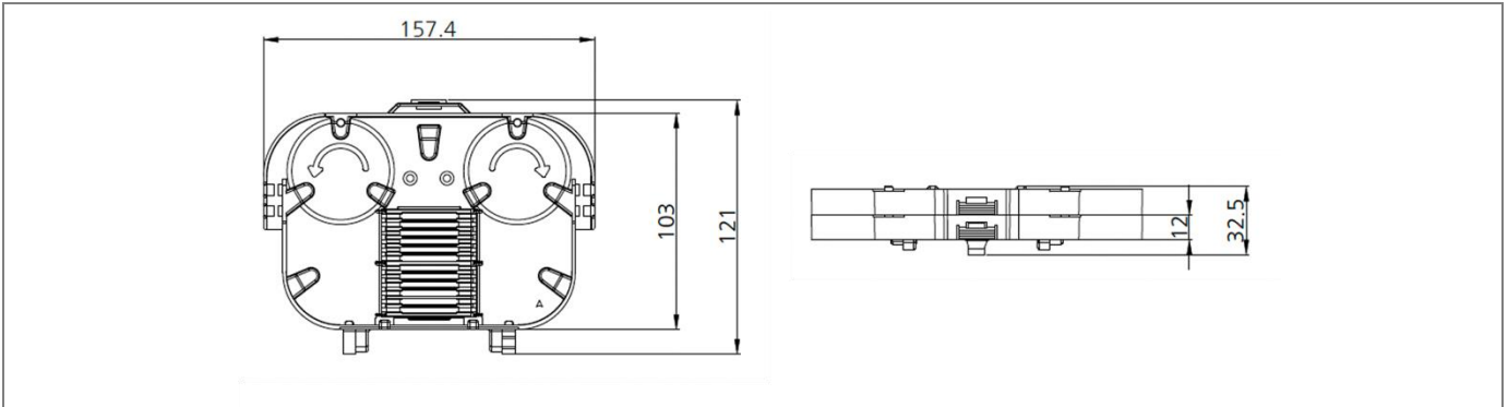
Khay hàn quang
